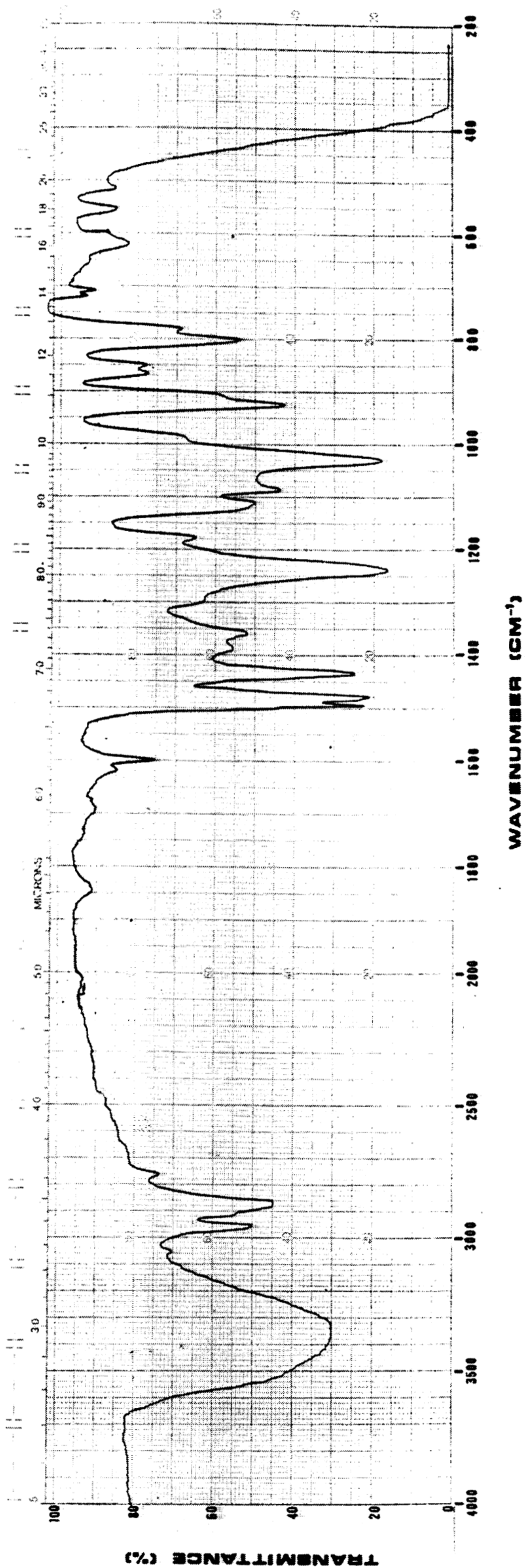
FIG. 4—IR spectrum of isosafrole glycol.
