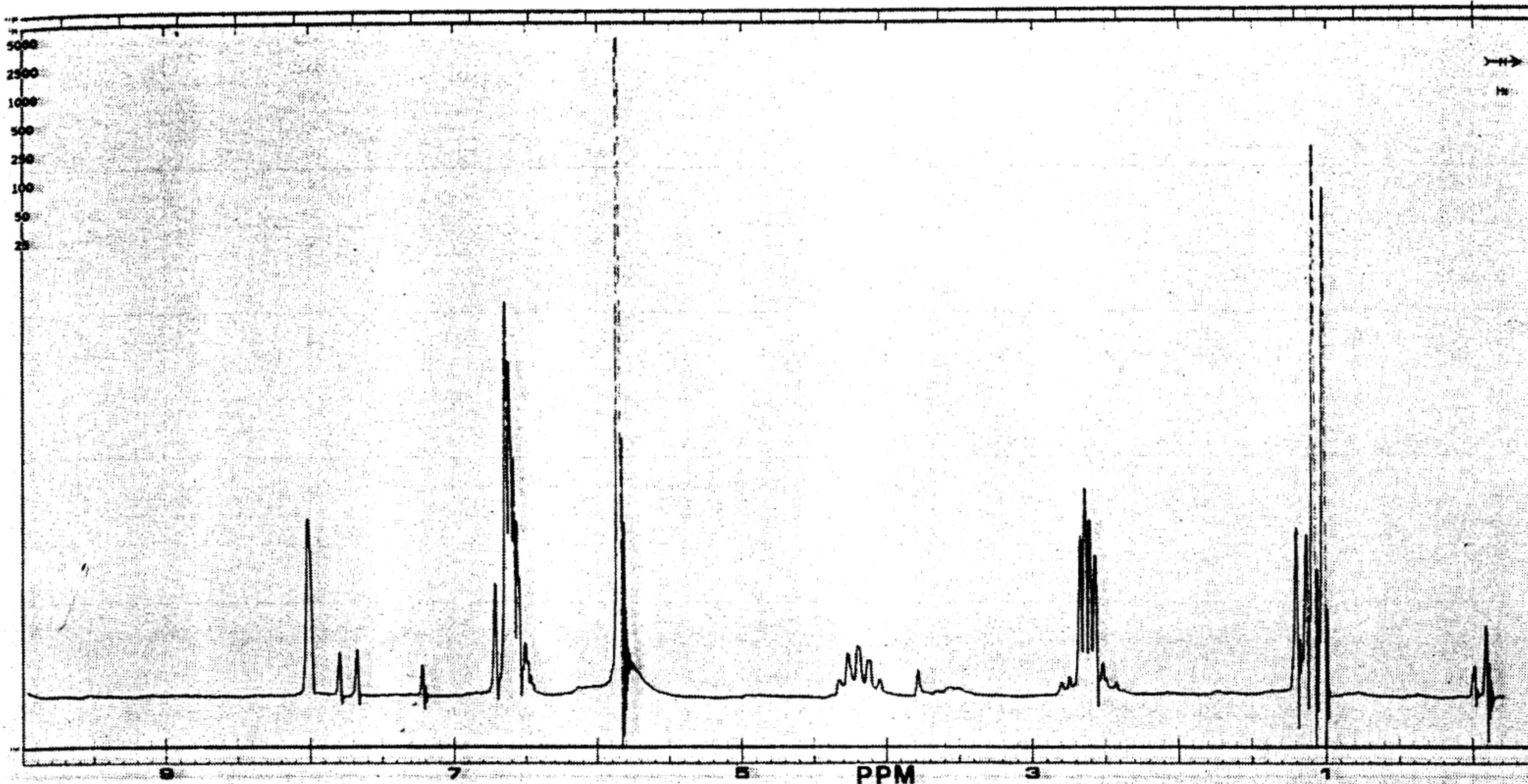
FIG. 11—NMR spectrum of N -formyl-MDA.
