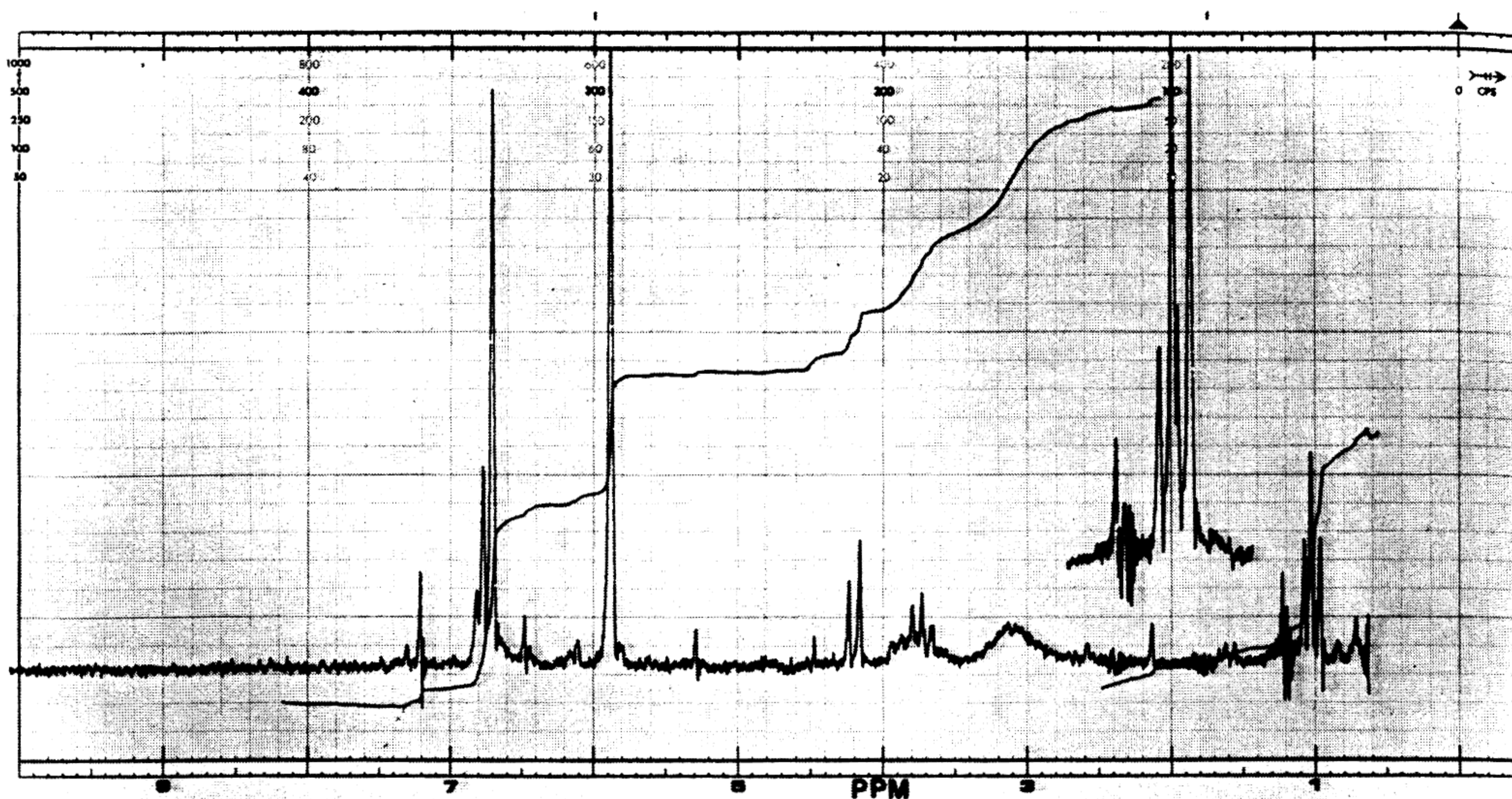
FIG. 5—NMR spectrum of isosafrole glycol.
