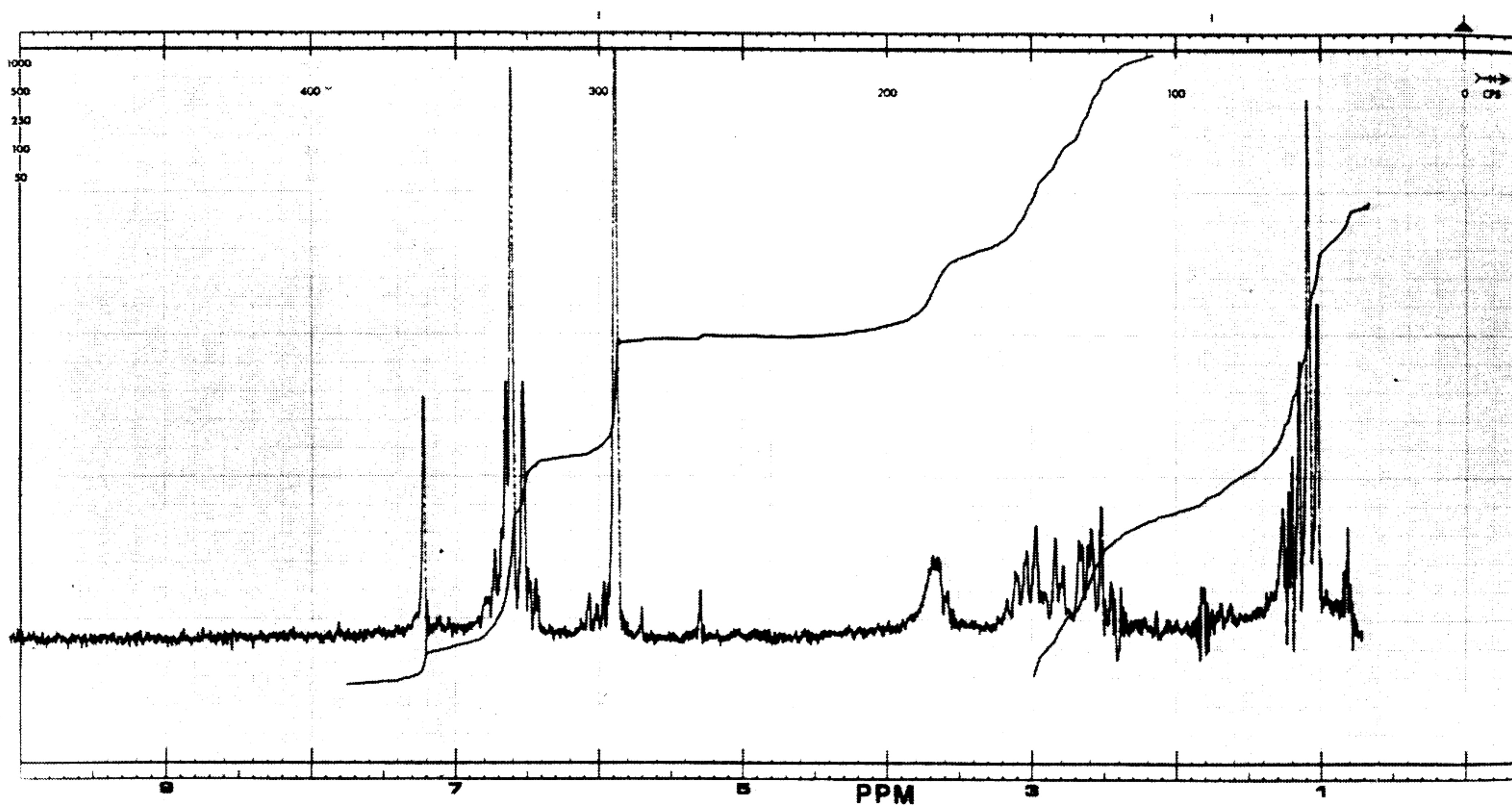
FIG. 14—NMR spectrum of di[1-(3,4-methylenedioxyphenyl)-2-propyl]amine.
