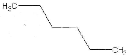
Hexane
