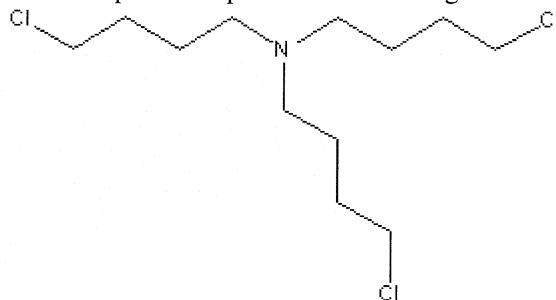
HN4
