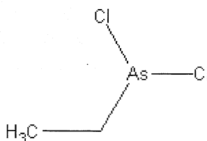
ED
