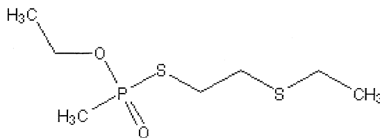
V-sub x
