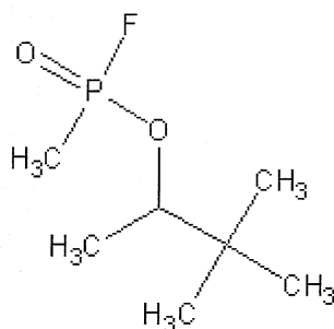
Soman
