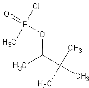
Chlorosoman
