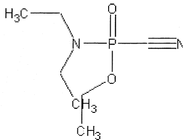
Tabun-II
