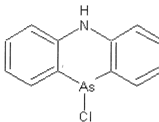
DM
