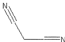
Malononitrile
