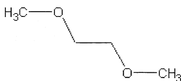
1,2-Dimethoxyethane
