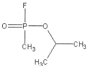
Sarin
