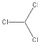
Chloroform
