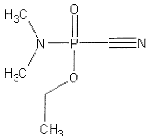
Tabun
