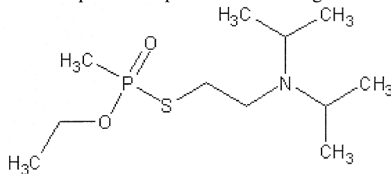
VX
