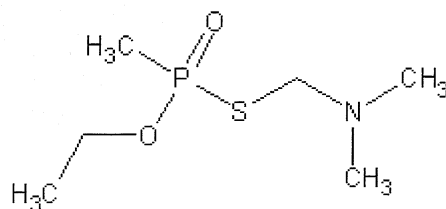
IIVX
